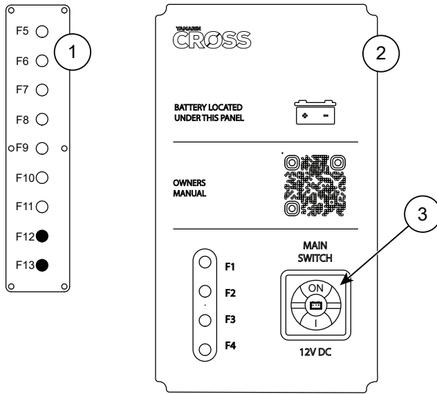
Figure 8.1 Cross 55 BR - Interrupteur principal et panneau de fusibles
