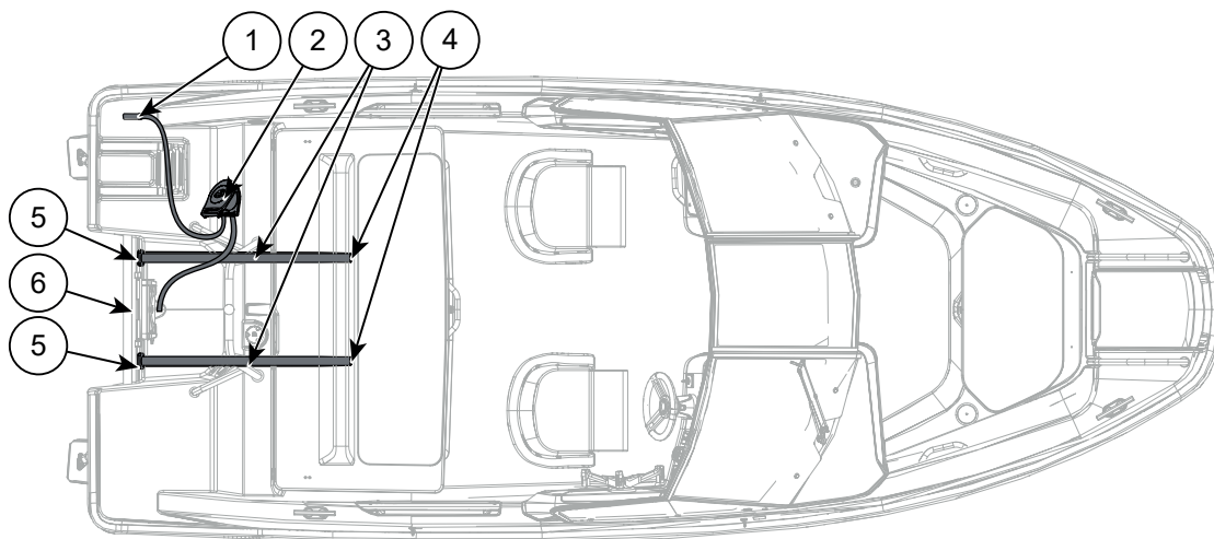
Figure 9.1 Cross 55 BR - Pompes et vidange de cale
