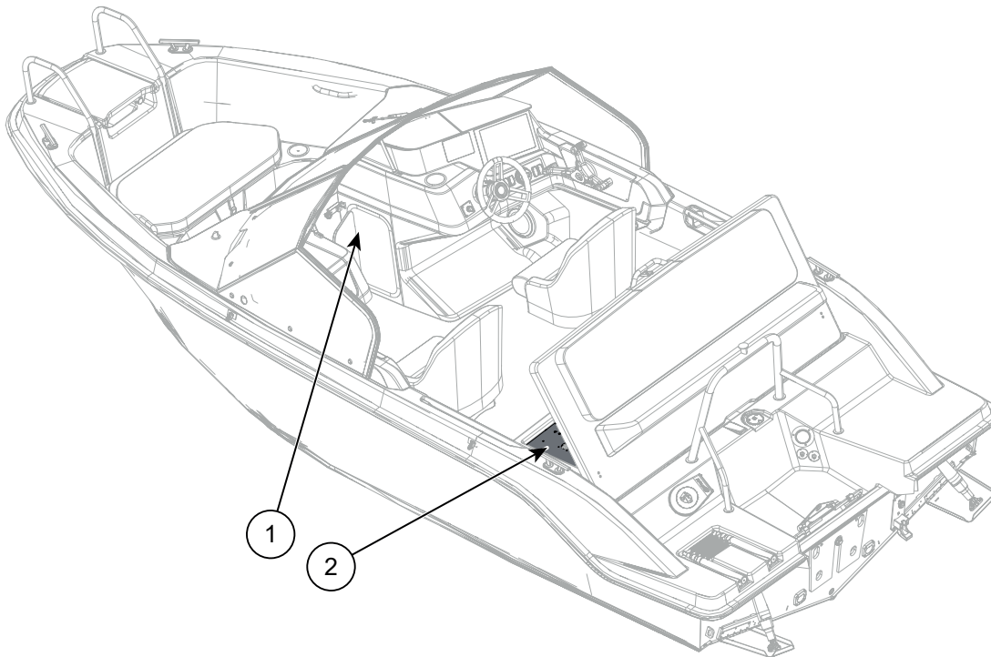
Figure 8.2 Cross 55 BR - Emplacement des panneaux de fusibles
