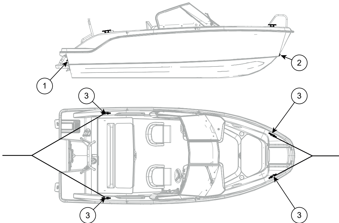
Figure 5.5 Cross 55 BR - Points d'amarrage et de remorquage
