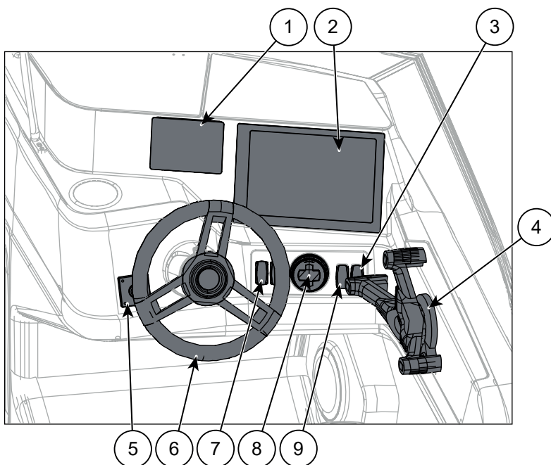
Figure 5.1 Cross 55 BR - Commandes du poste de barre
