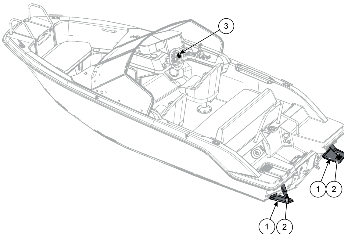
Figure 5.4 Cross 55 BR - Système de trim
